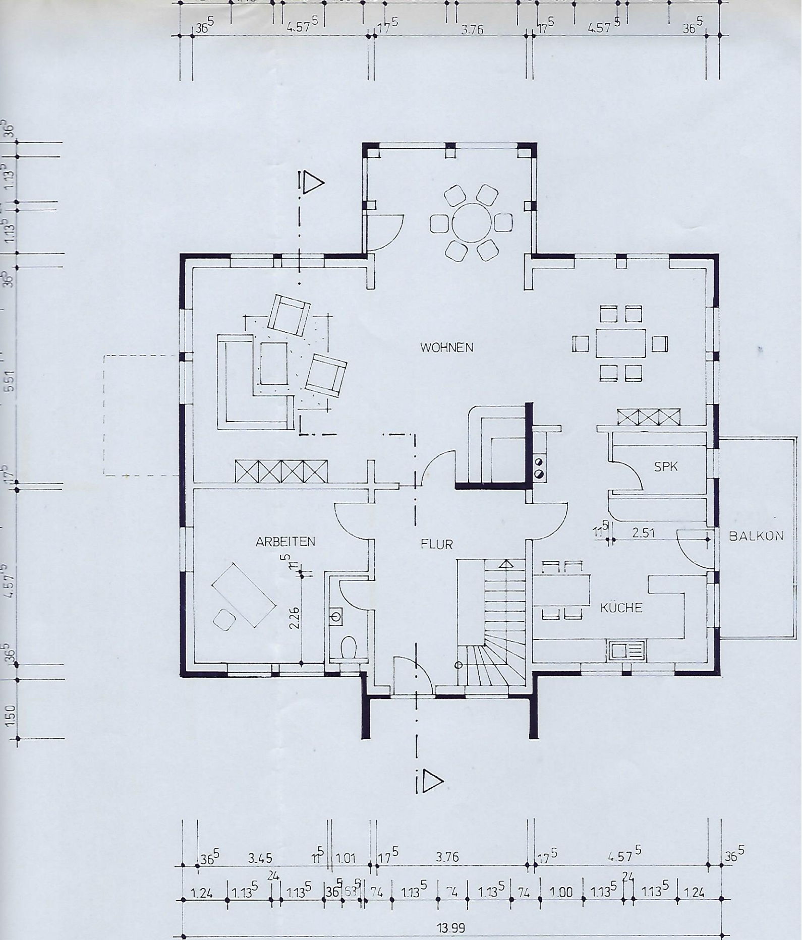
ERDGESCHOSS
